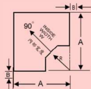
90 度
