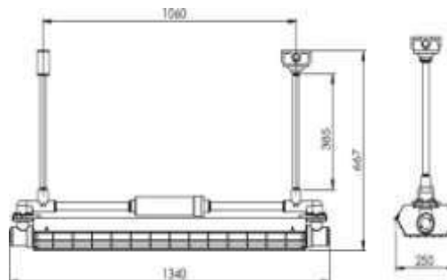
吊管型
