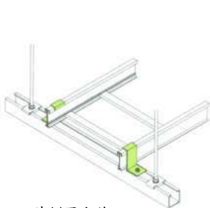
外側固定片
