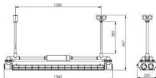
吊管型
