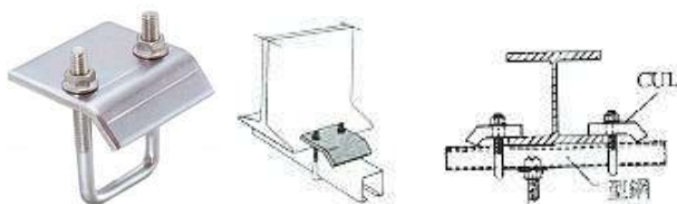
型鋼用直角管束 RAC
