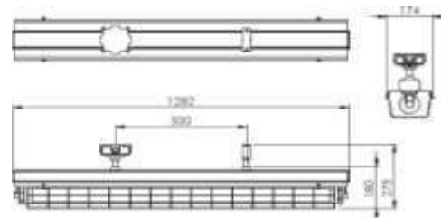
吊管型
