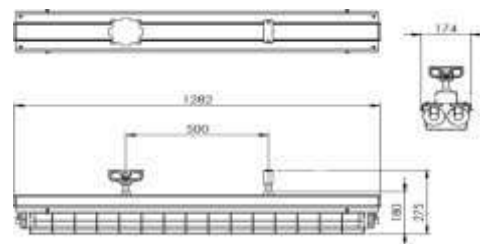
吊管型
