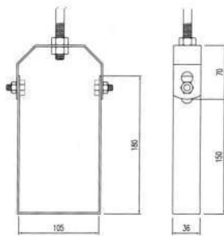
燈用線槽門型吊架
