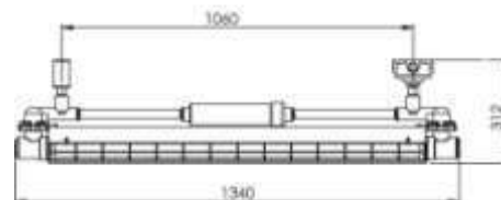
吊管型
