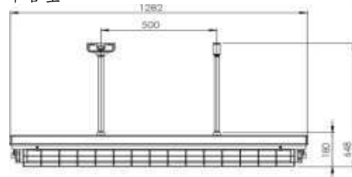
完全吸頂型
