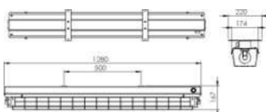
完全吸頂型
