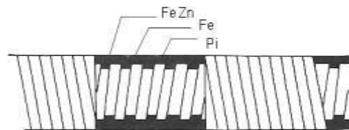
PZ-4 JIS C 8309
