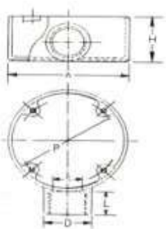
氣密燈穿線匣 GH 型
