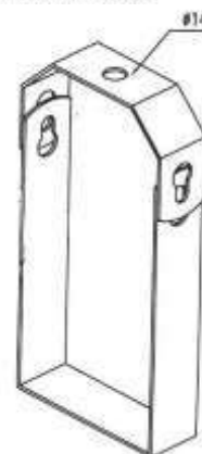
燈用線槽門型吊架
